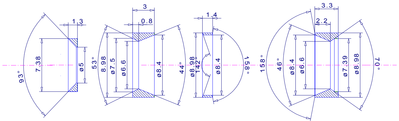
n71131,2,3,4 pierścienie UWAGA: wszystkie pierścienie zaokrąglić 0.2
